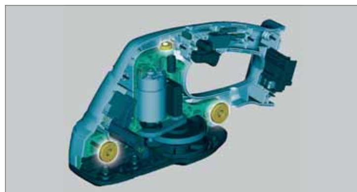
Antivibrační úprava stroje
